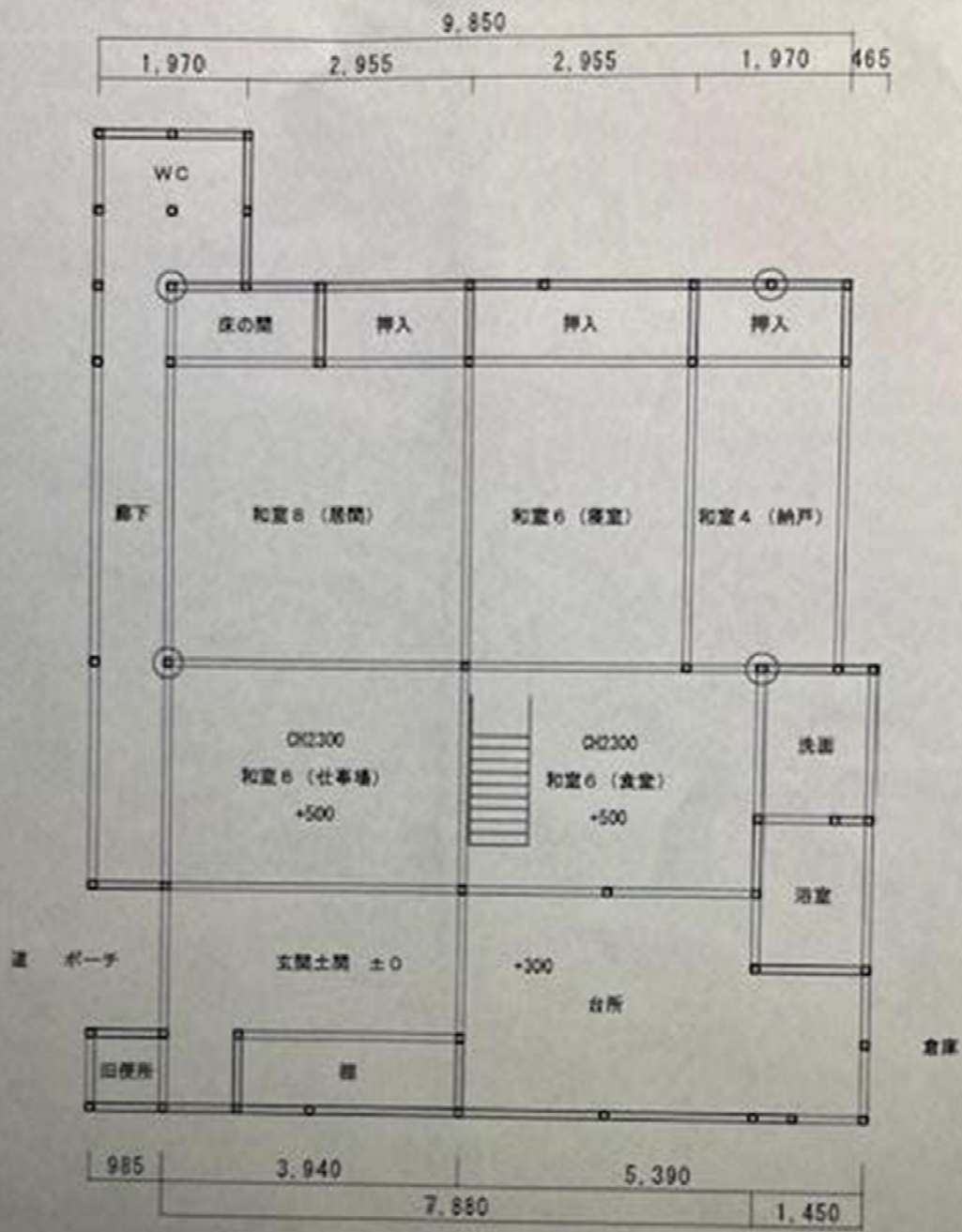
1 階平面図
