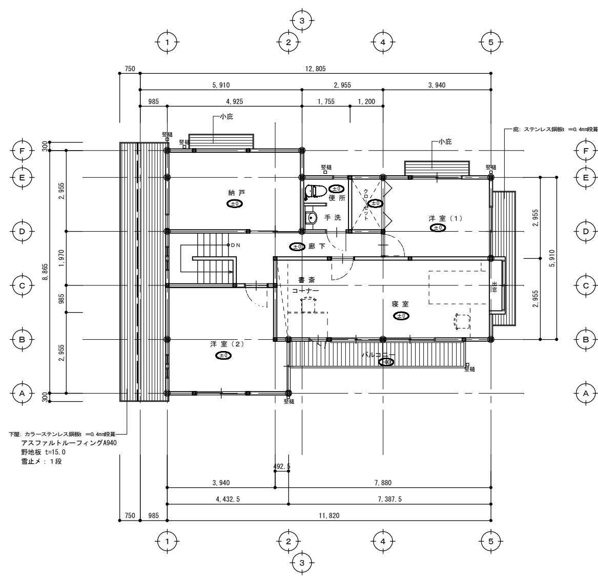
2 階 平 面 図
